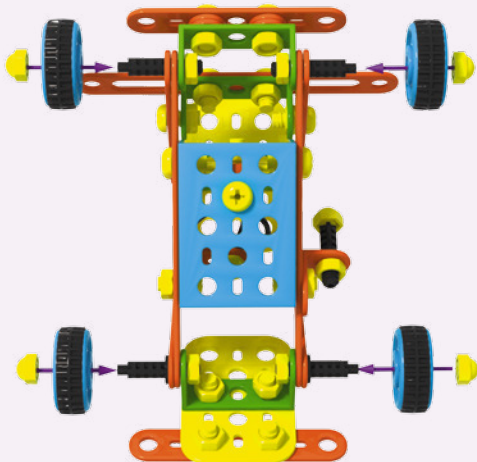
Установка колёс
