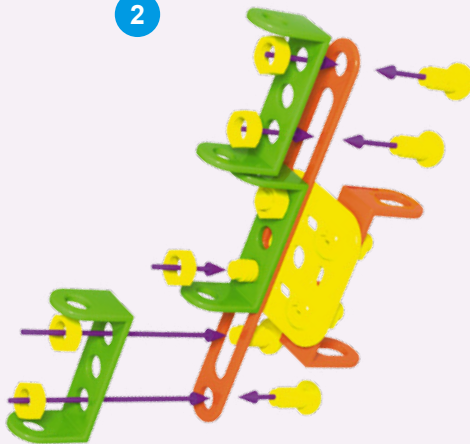
Сборка ножа
