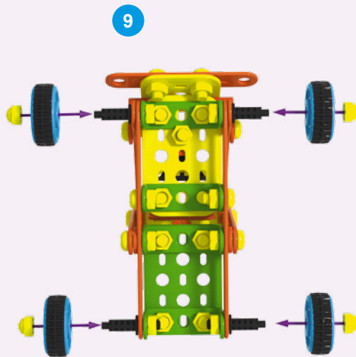
Установка колёс
