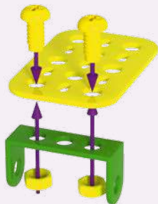
Сборка кабины
