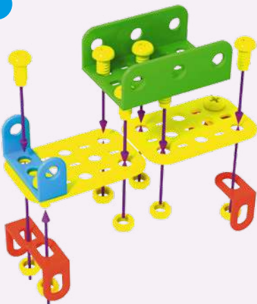
Сборка рамы
