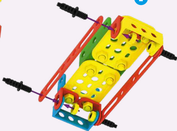
Сборка рамы (2 этап)
