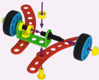
Крепление шасси
